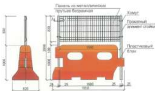
Рисунок А.8 - Фрагмент сечения сигнального временного ограждения
